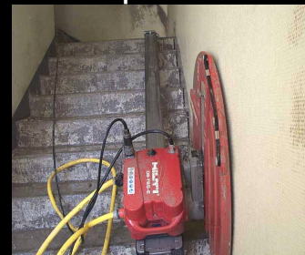
Découpe d'escalier
